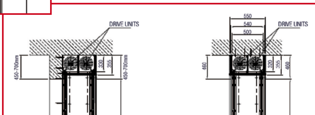
Sous dalle Béton
