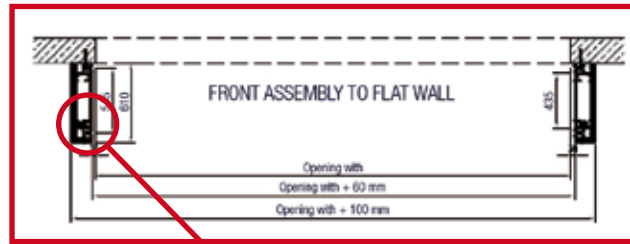
Pose en applique
